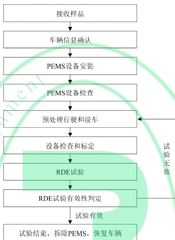
图 1 RDE 型式检验流程图
