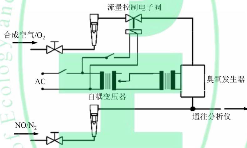
图 A.1 \text{NO}_x 转化器效率试验装置
