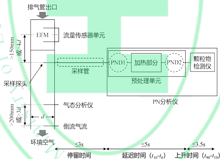
图 A.2 PN 分析仪构造原理的例图
