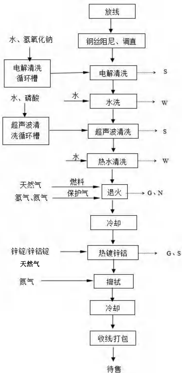
图 3.9-1 热镀锌（铝）生产线工艺段工艺流程及排污节点图
