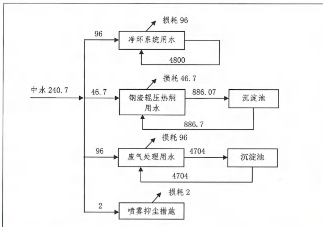
图 3.4-1 项目水平衡图（单位：m 3 /d）
