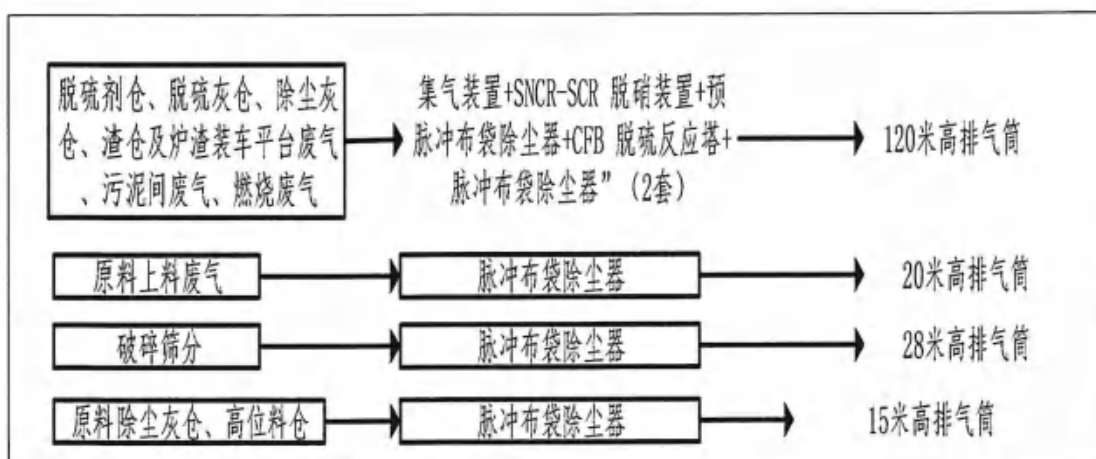
图 4.1-2 废气治理示意图
