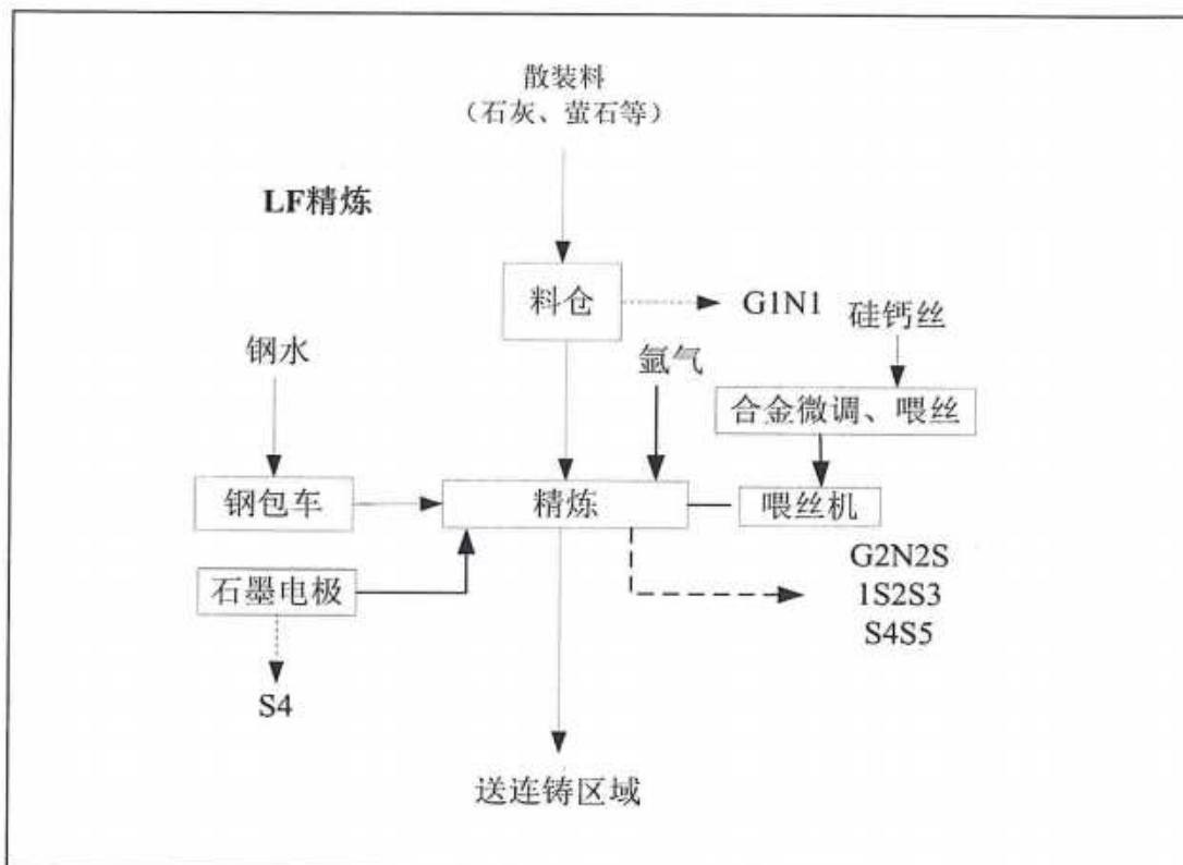
图 3.5-1 生产线工艺流程图
