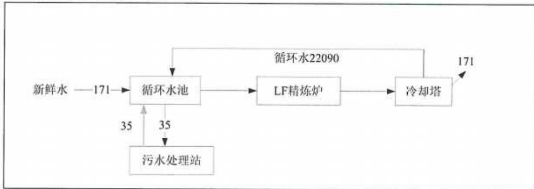
图 3.4-1 项目水量平衡图 单位 m 3 /d
