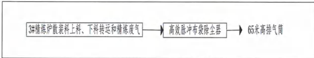
图 4.1-2 废气治理示意图
